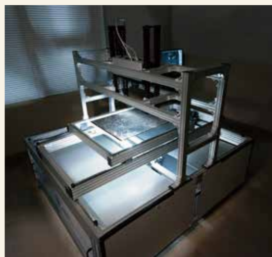
ガラス乾板専用超高精細スキャナー
